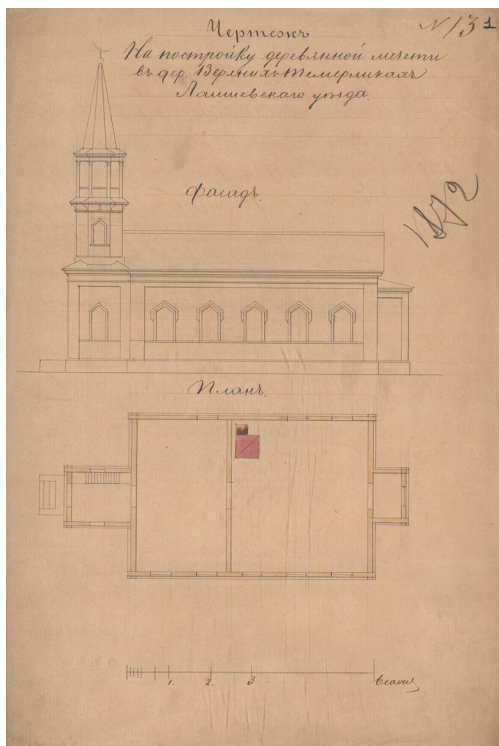
Агач мәчетнең фасады һәм планы. 1872 ел. Татарстан Республикасы Дәүләт архивы, 2 ф., 2 тасв., 273 эш, 1 кз.
