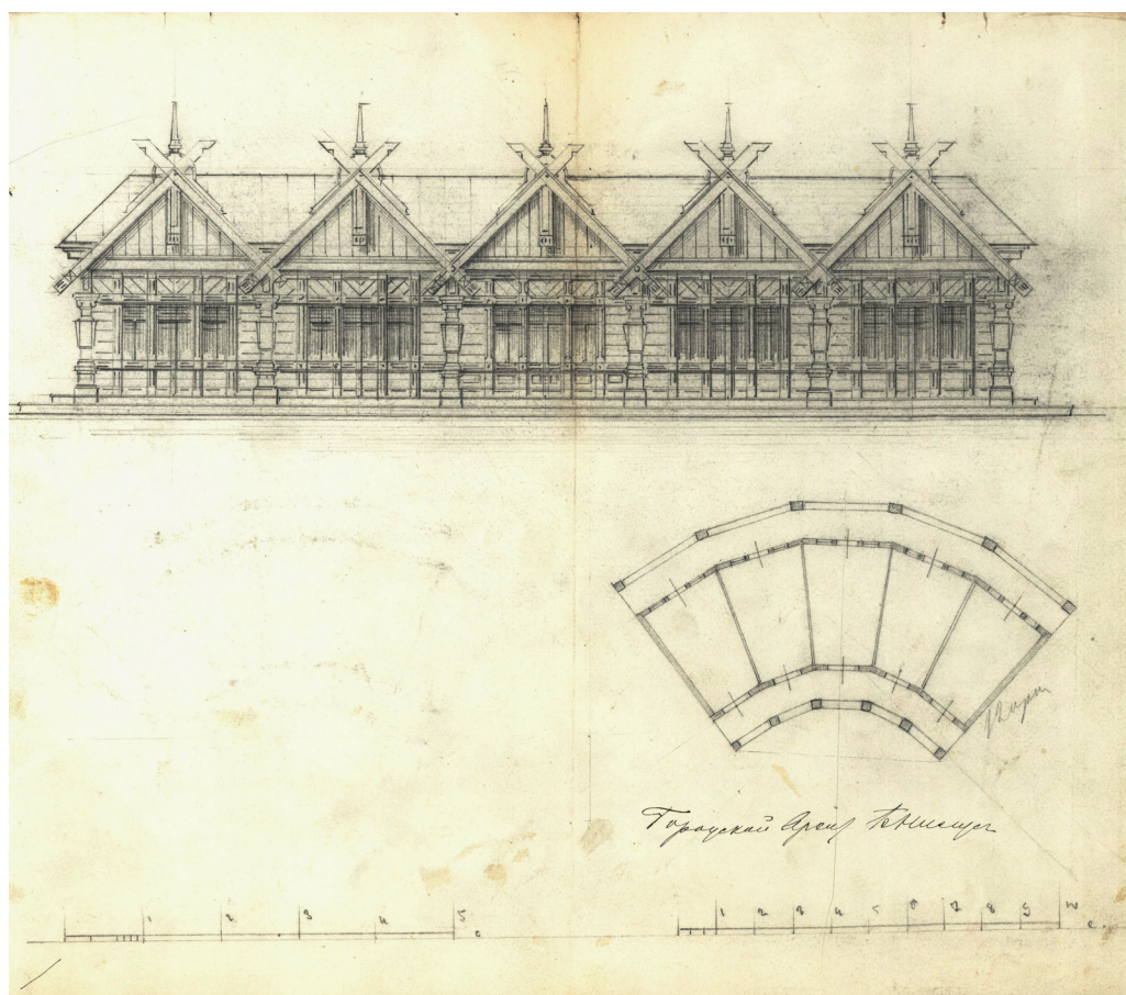
План фасада лавок на Сенной площади. ГА РТ, ф. 98, оп. 3, д. 1968, л. 3.
